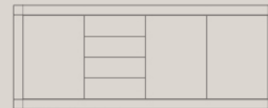
BER DRES 4 DLDD B 2170 mm / H 860 mm / D 530 mm
